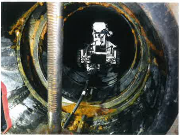
八千代幹線(下流側)の調査状況
