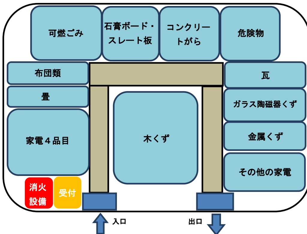
図表 3-12 一次仮置場の分別配置の例
