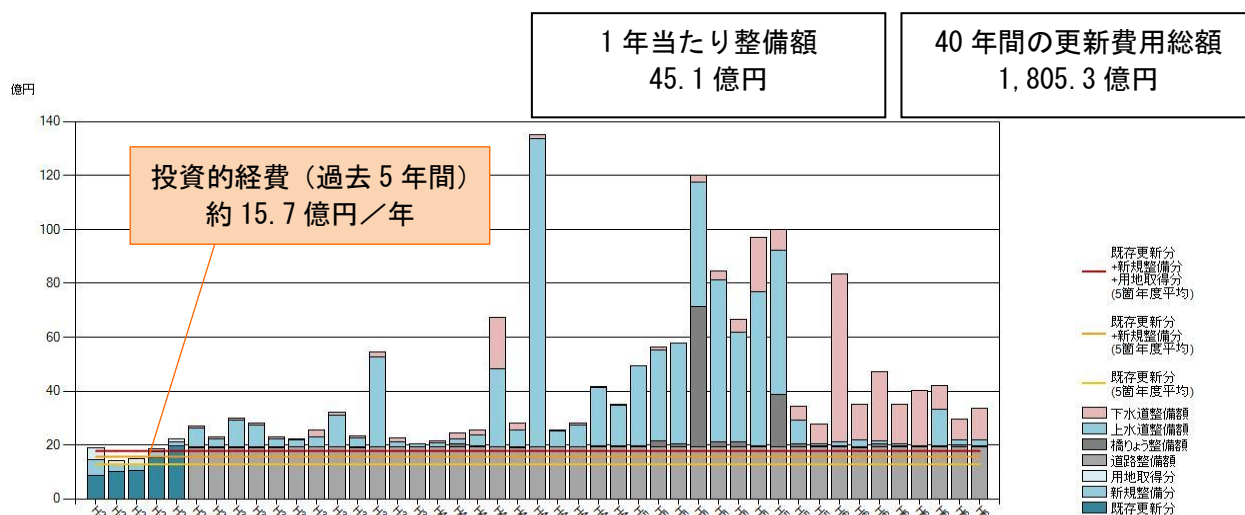
図表 25 インフラ資産の将来の更新等費用の推計 公共施設等更新費用試算ソフト
