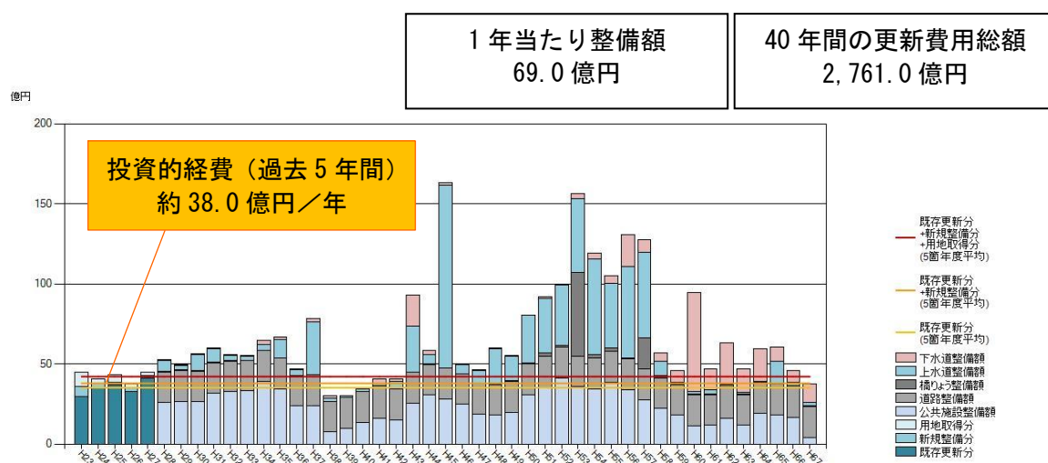
図表 26 公共施設とインフラ資産の更新等費用推計 公共施設等更新費用試算ソフト
